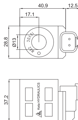
Model:LC9-08-S-*DR(25W) DEUTSCH CONNECTOR
