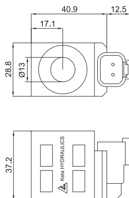
Model:LC2-08-S-*DR(16W) DEUTSCH CONNECTOR
